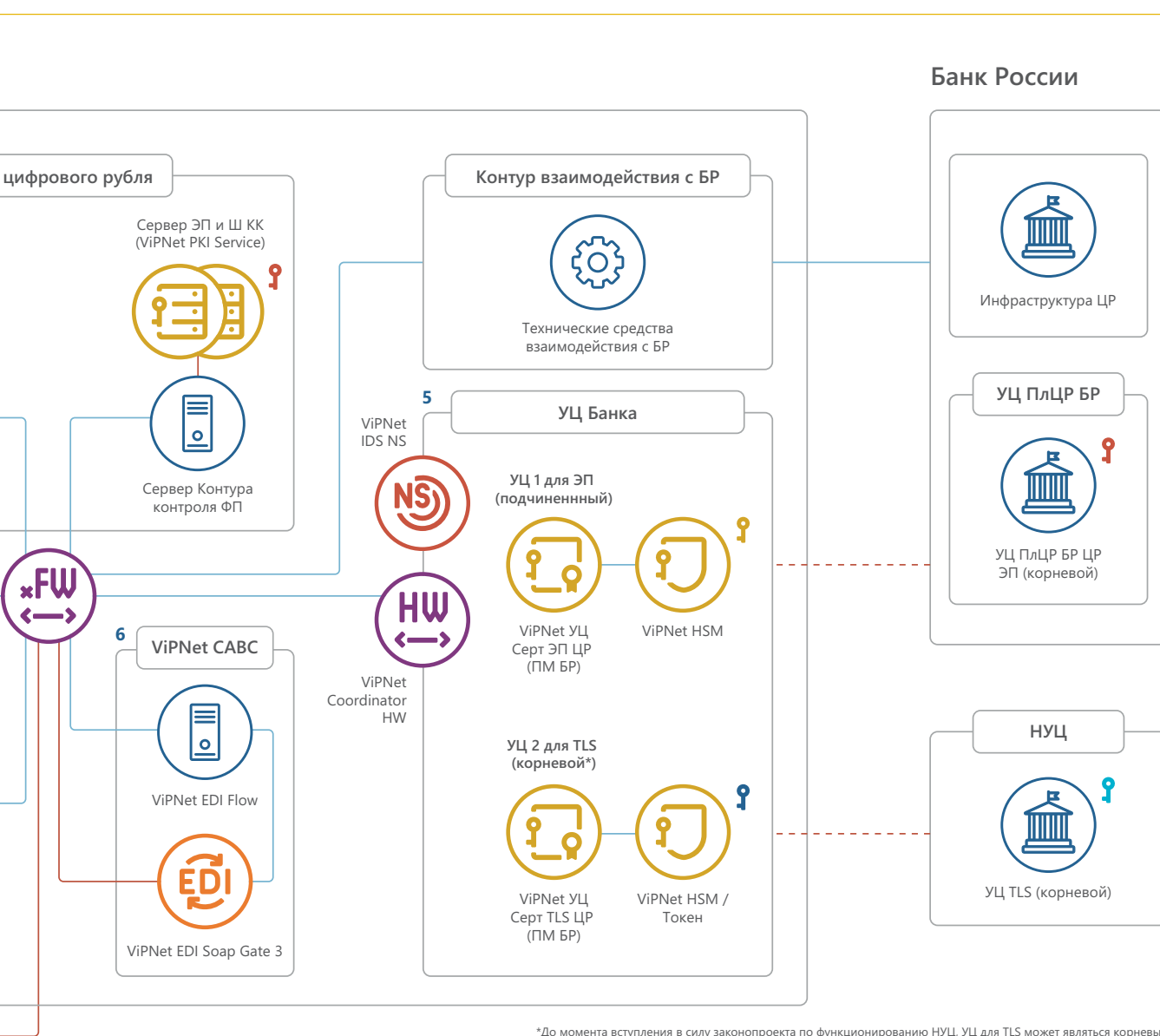
Схема 3. Предполагаемая схема защиты инфраструктуры платформы цифрового рубля
